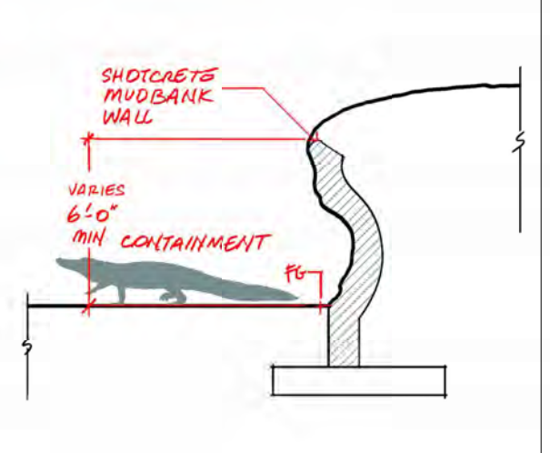
8 F1 - Alligator Mud Bank - Section 1/2" = 1'-0"
