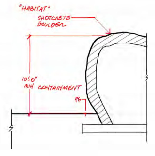
2 G2 - Cheetah Rockwork - Section 1/2" = 1'-0"
