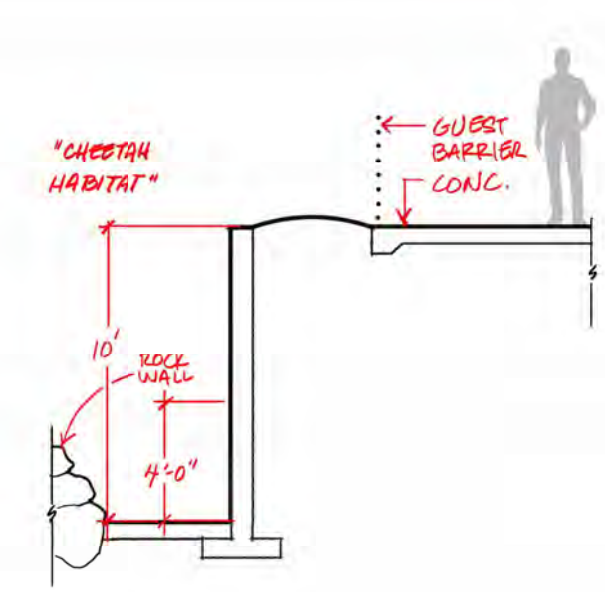
3 G3 - Cheetah CIP Wall - Section 1/2" = 1'-0"
