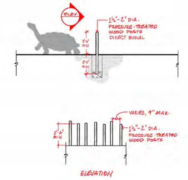
6 D2 - Tortoise Reed - Section 1/2" = 1'-0"
